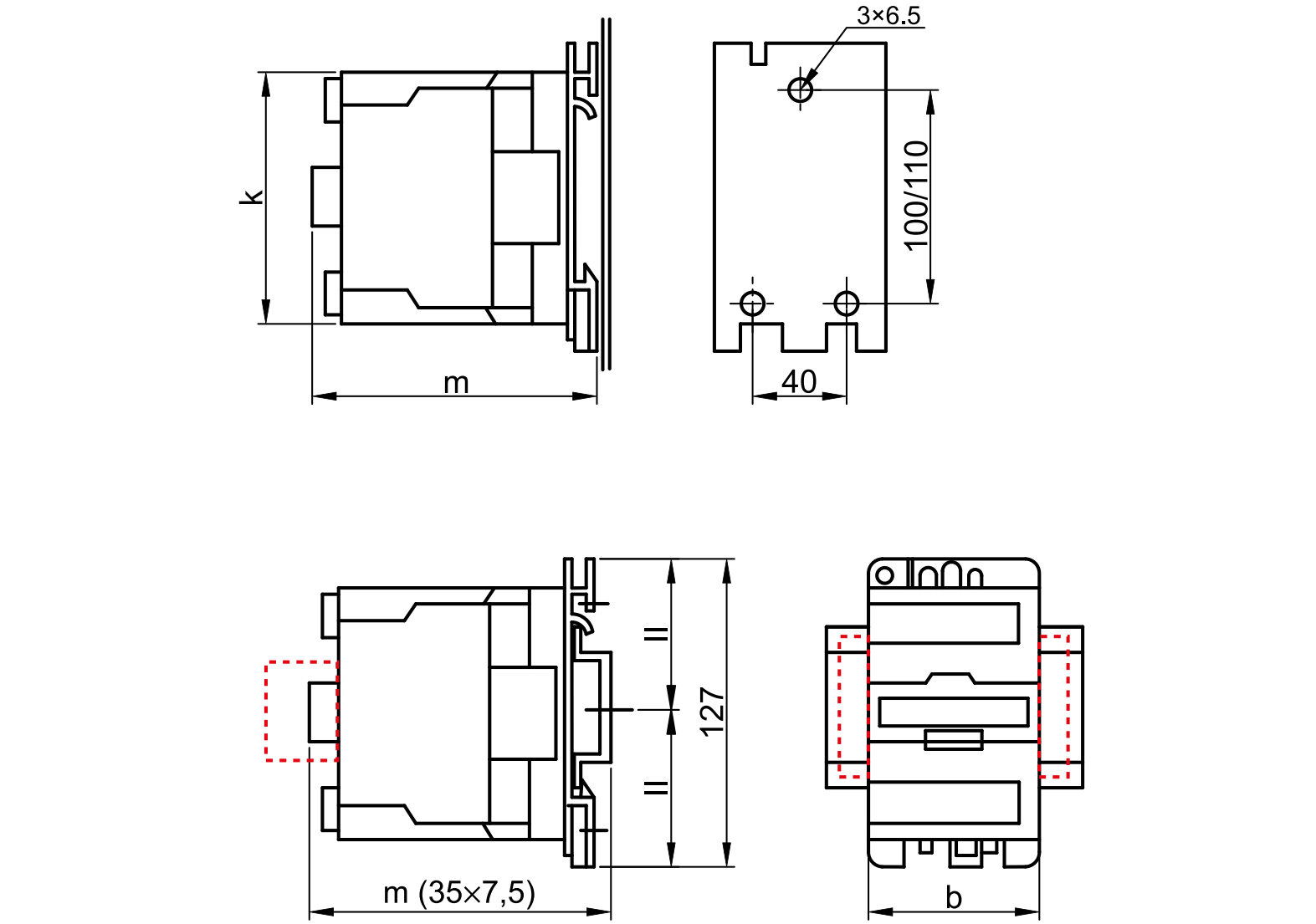
Rozmerový výkres
